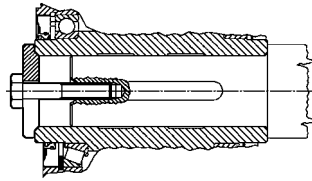
Stirnrad und Kegelschneckenrad Größe MR 31 63
