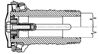
Stirnrad und Kegelschneckenrad Größen 180 ... 360
