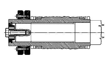
Stirnrad und Kegelschneckenrad Größe 400 ... 6301
