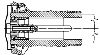
Stirnrad und Kegelschneckenrad Größe 180 ... 360
